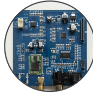
HDMI, BT ve Dijital Dikkatli Şekilde Ayrılmış Özel Lineer Güç Kaynağı
